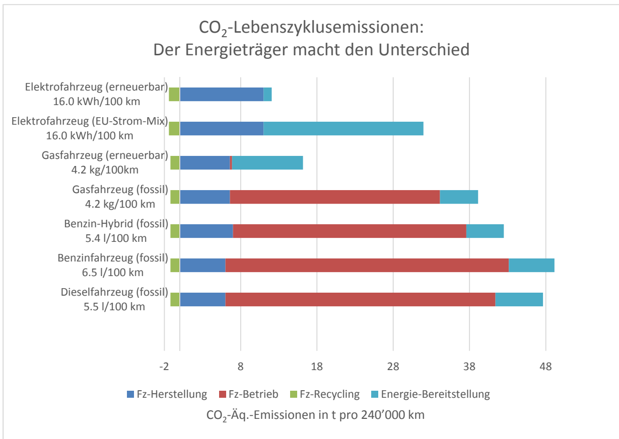
Abbildung 1: Treibhausgasbilanz von Personenwagen – Vergleich verschiedener Antriebskonzepte
