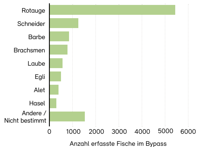
Abb. 49: Anzahl Fischnachweise im Bypass während der Wirkungskontrollen
