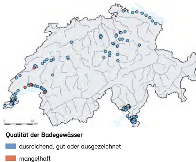
Abb. 13: In der Schweiz kann fast überall bedenkenlos gebadet werden
