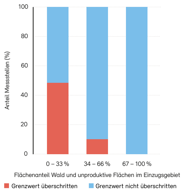
Abb. 10: Je geringer der Flächenanteil Wald und unproduktive Flächen im Einzugsgebiet einer Messstelle, desto höher sind die DOC-Konzentrationen
