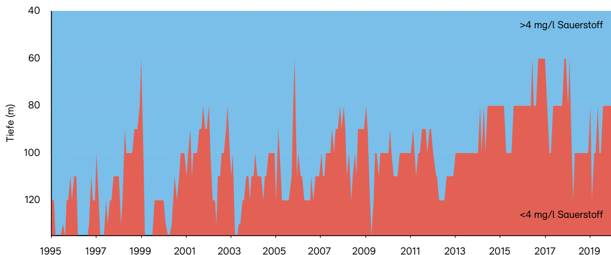
Abb. 32: Wärmere Seewasser führt zu einer Abnahme der Durchmischungstiefe im Zürichsee, wodurch sich die sauerstoffarme Zone ausdehnt
