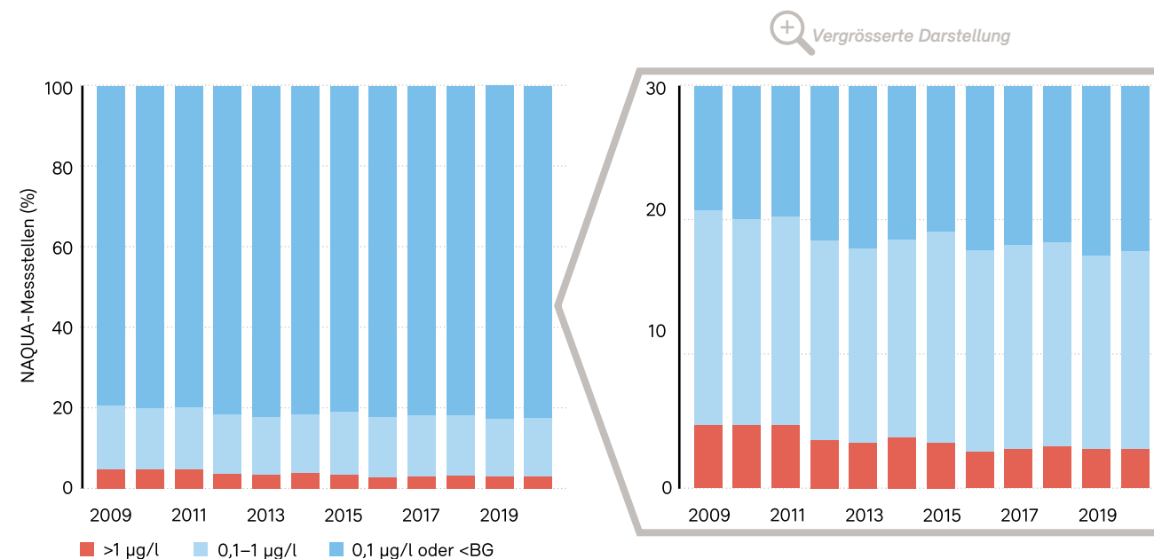
Abb. 7: Die Grenzwertüberschreitungen durch flüchtige halogenierte Kohlenwasserstoffe (FHKW) im Grundwasser gingen in den letzten Jahren auch dank der Sanierung belasteter Standorte leicht zurück BG: Bestimmungsgrenze.
