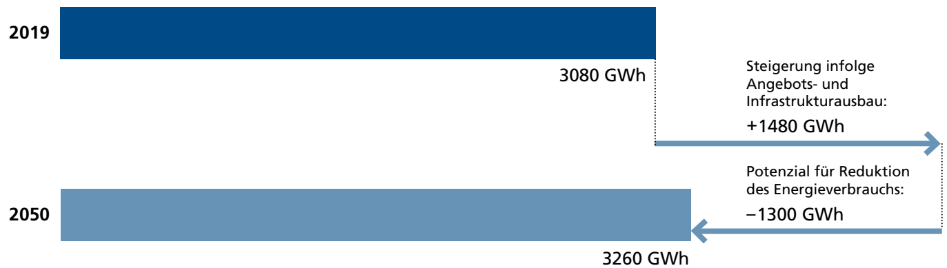
Abbildung 12 Gesamtenergiebedarf des Bahnsystems und Einsparpotenzial (Quelle: SBB 2021c)
