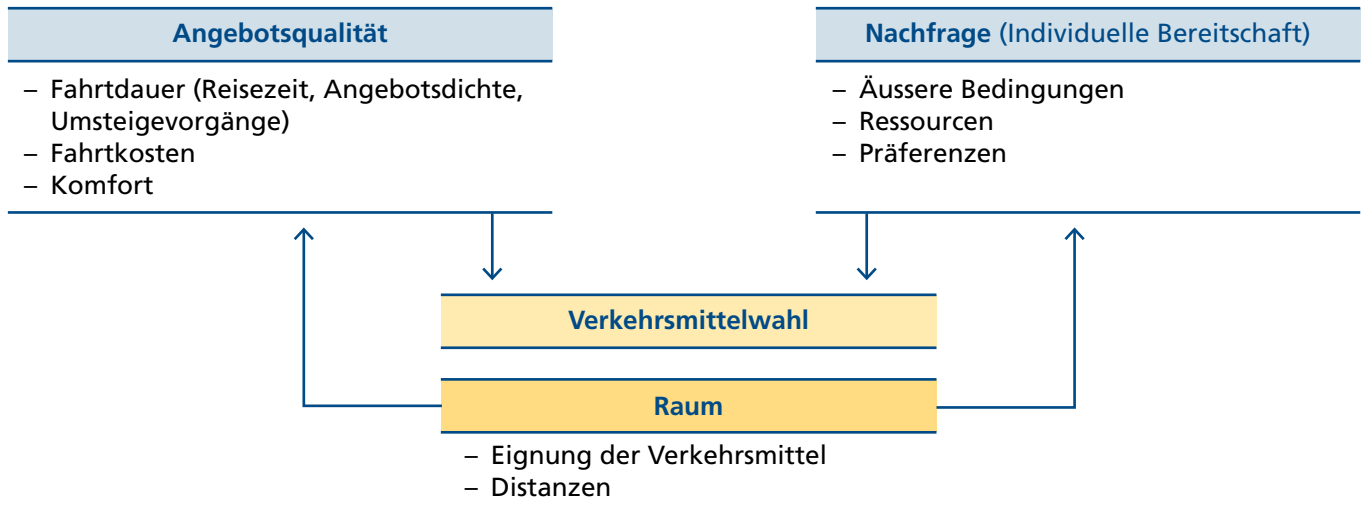
Abbildung 6 Einflussfaktoren für die Verkehrsmittelwahl (Quelle: 6t-bureau de recherche 2019, Darstellung: BAV)
