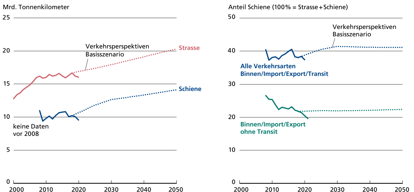
Abbildung 5 Verkehrsleistung und Modal-Split im Schienengüterverkehr (Quelle: BFS, ARE 2021; Darstellung: BAV)
