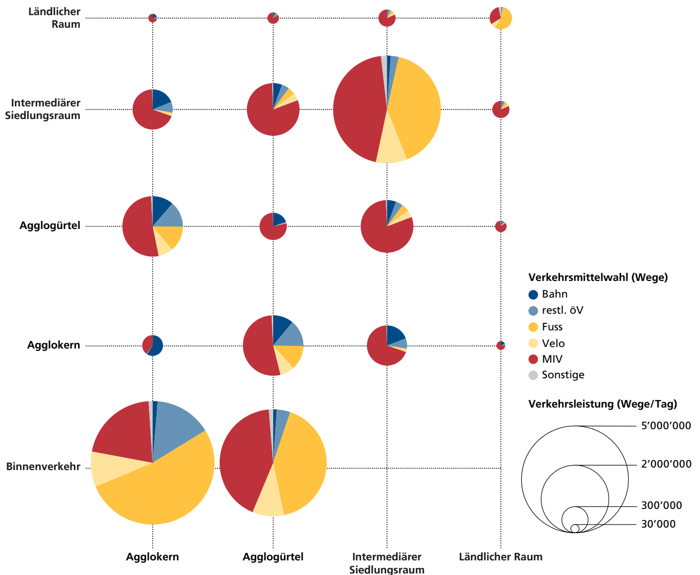
Abbildung 7 Mobilitätsverhalten nach Raumtypen, 2017, Verkehrsaufkommen in der Schweiz und Modalsplit nach Wegen, Auswertung für gesamte Schweiz (Quelle: Metron 2021)
