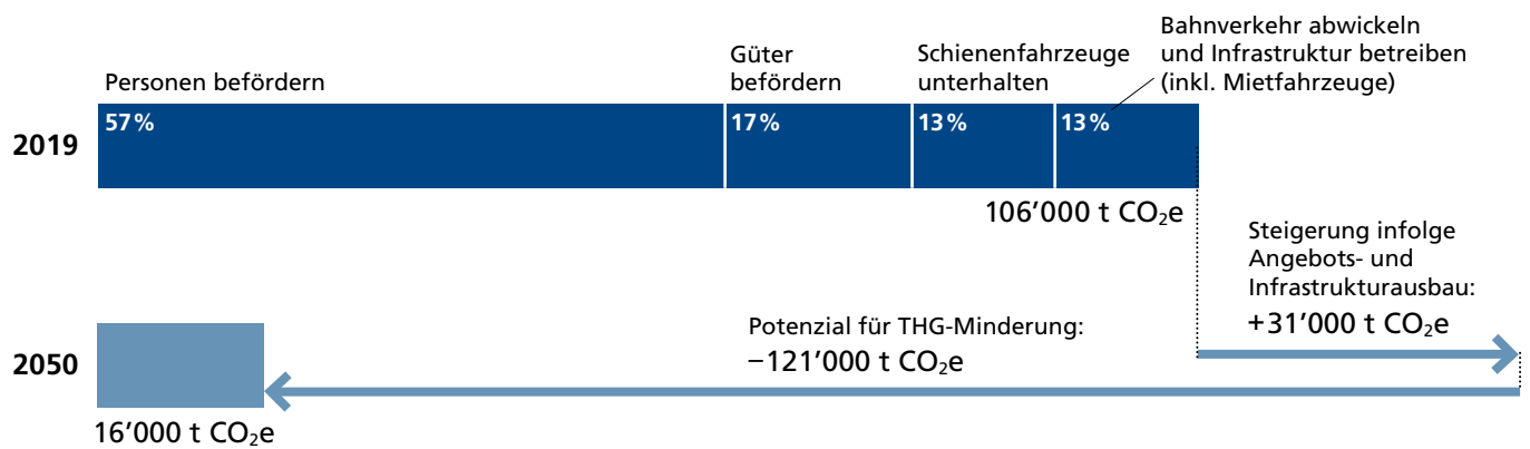
Abbildung 11 Direkte THG-Emissionen des Bahnsystem und Potenziale für THG-Minderungen (Quelle: SBB 2021c)
