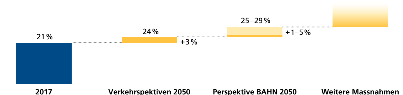
Abbildung 8 Verlagerungspotenzial im nationalen Personenverkehr (Quelle: SBB 2021a, SMA 2021; Darstellung: BAV)
