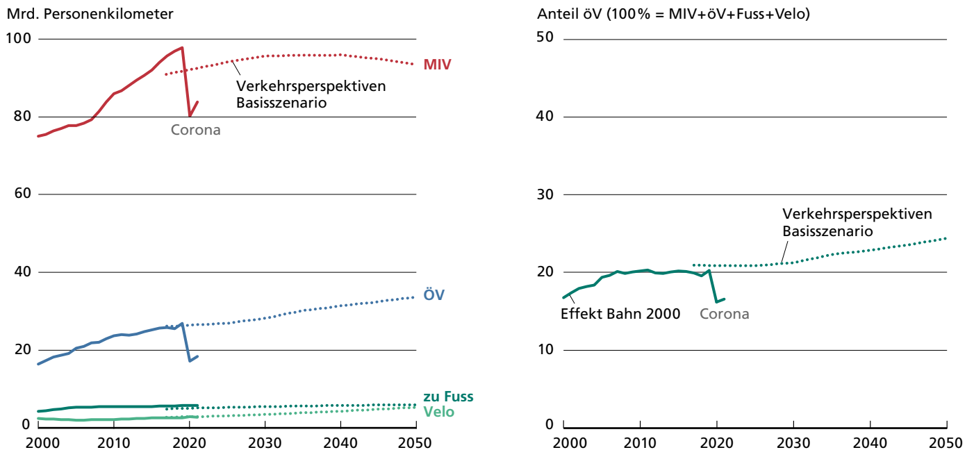
Abbildung 4 Verkehrsleistung und Modal-Split öV im Personenverkehr (Quelle: BFS, ARE 2021; Darstellung: BAV)
