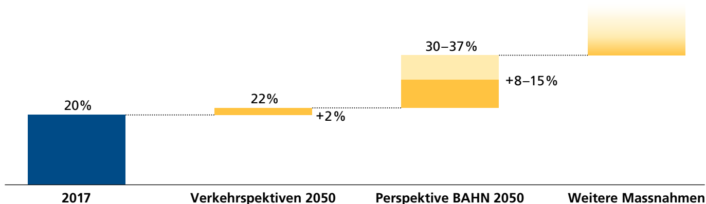
Abbildung 10 Verlagerungspotenzial im Güterverkehr (Binnen-, Import- und Exportverkehr) (Quelle: SBB 2021b, EBP 2021)
